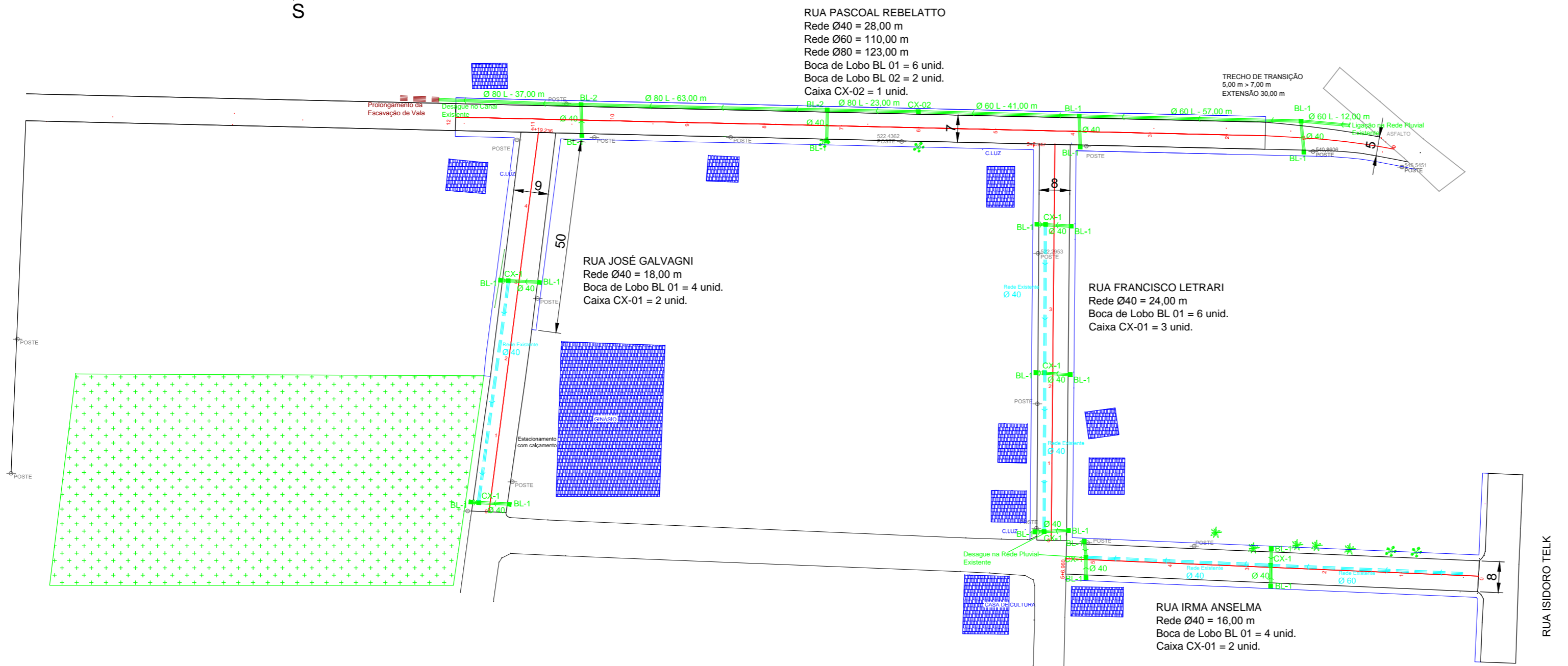
PLANIMÉTRICO ESC.: 1/1000
