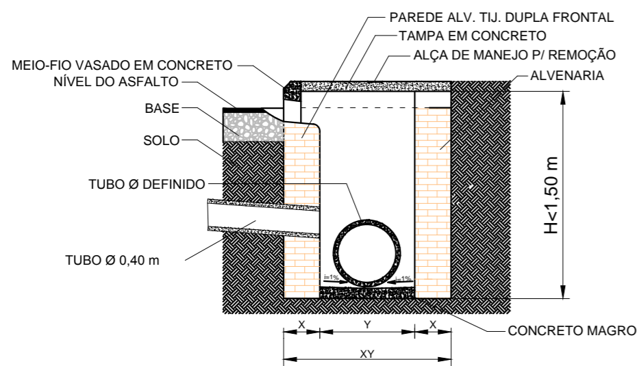
SEÇÃO TRANSVERSAL A.A
