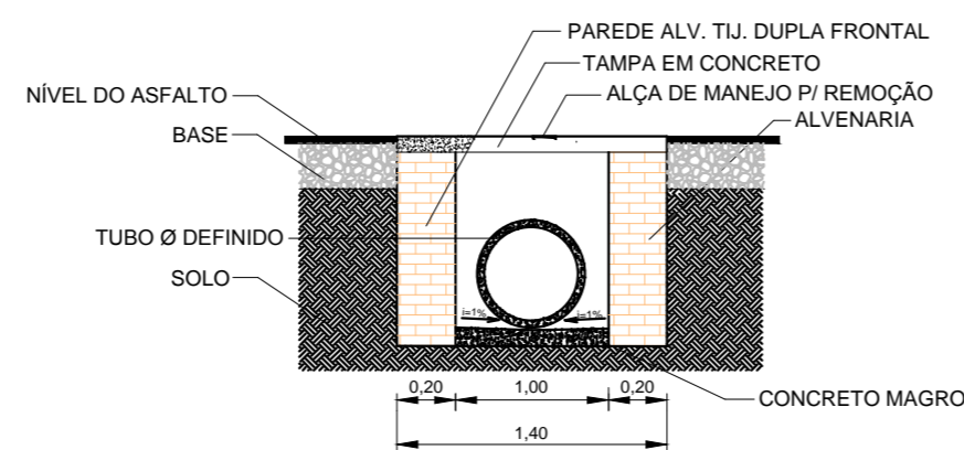
SEÇÃO TRANSVERSAL A.A
