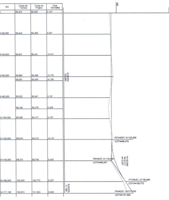
PERFIL LONGITUDINAL - FRECHO 02
