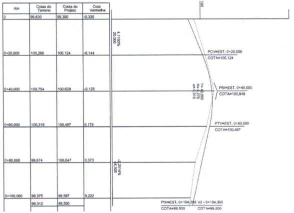
PERFIL LONGITUDINAL - FRECHO 01
